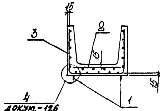
СХЕМА АРМИРОВАНИЯ
